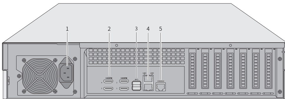
图1-4 TL-TUMS2600-N-A后面板示意图
