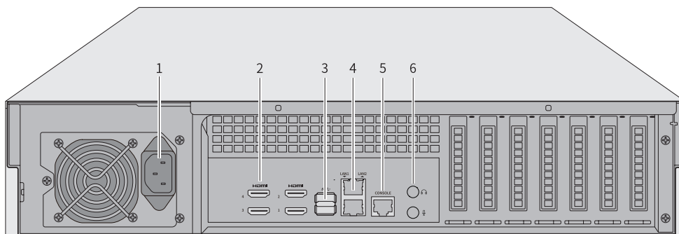
图1-3 TL-TUMS2500-N-A后面板示意图
