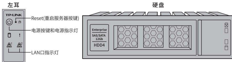
图1-2 前面板按键与指示灯
